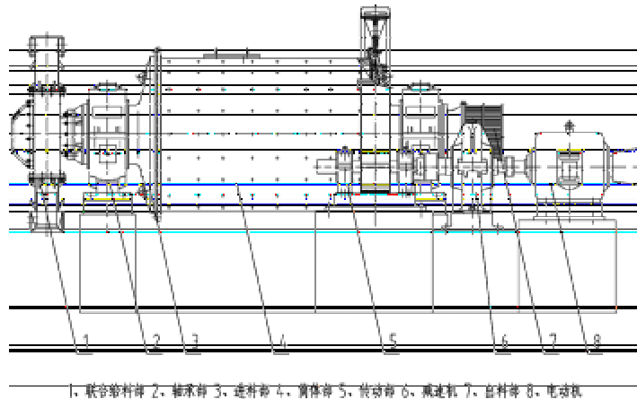
1. 联合给料器 2. 轴承座 3. 进料器 4. 筒体 5. 传动轴 6. 减速机 7. 出料器 8. 电动机
